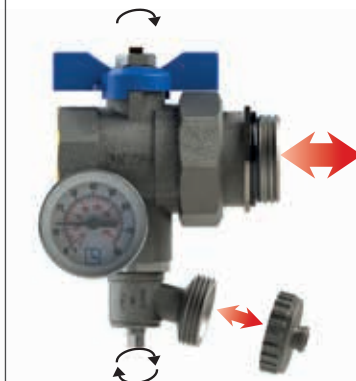
VALVOLA CARICO / SCARICO ACQUA
