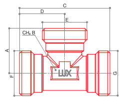
RT 911 Raccordo a T.
