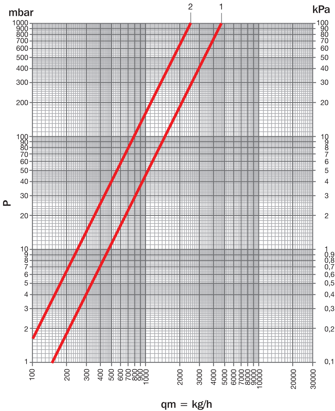
DIAGRAMMA DI PORTATA
